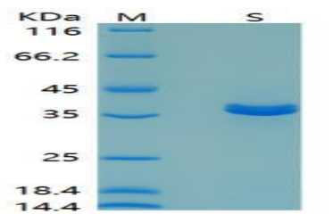
SDS-PAGE Result
