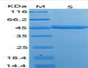
SDS-PAGE Result
